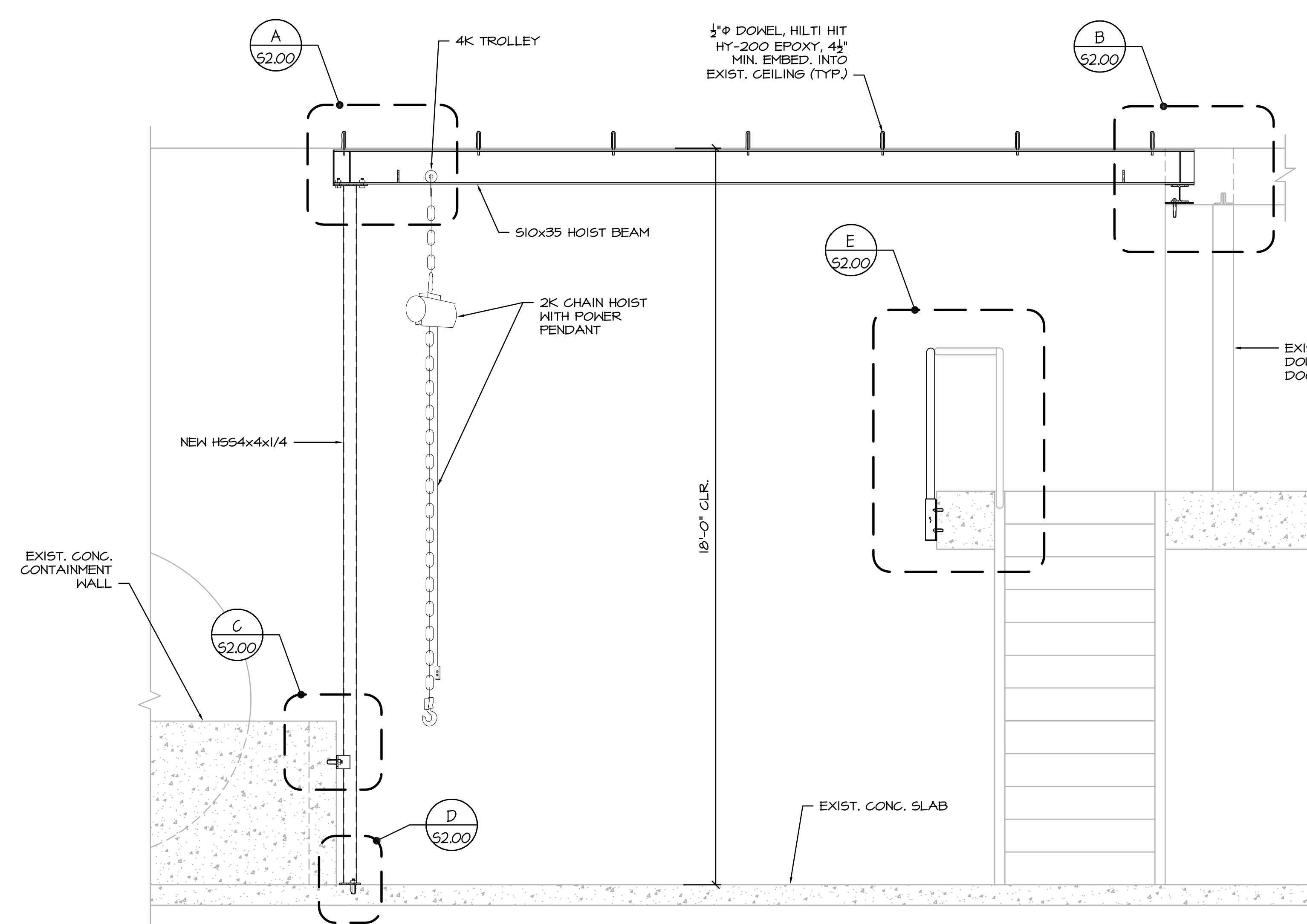
ELEVATION SCALE: 1/2"=1'-0" (1) 51.00
